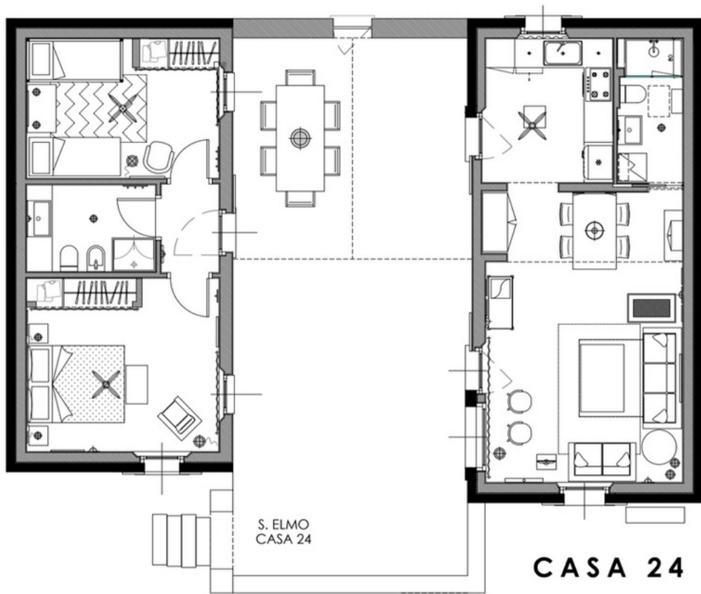
S. ELMO CASA 24 - Pianta piano terra 1: 50 - architetto Laura Sonzogni_2017
