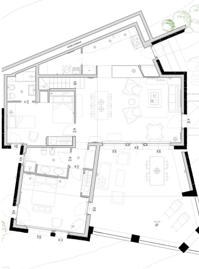
CASA 8 - Pianta piano terra 1: 50 - arch. Laura Sonzogni_ ARREDO 2013
