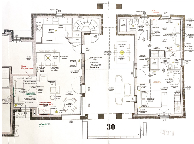
30 CASA 30 - Pianta piano terra 1:50 - arch. Vito e Laura Sonzogni_20.03.2014
